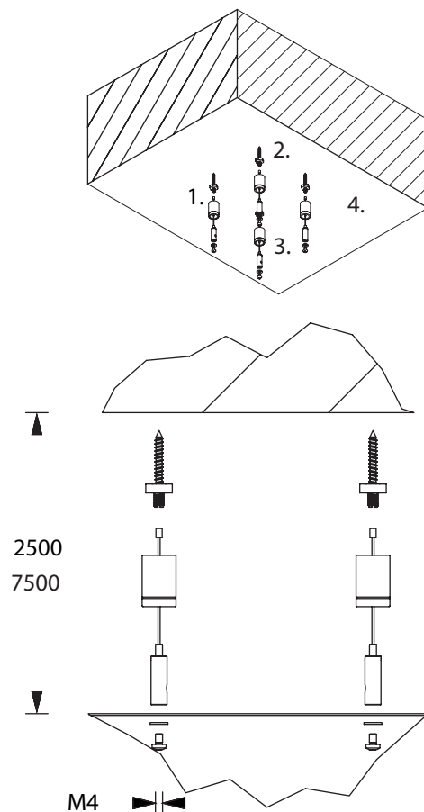
1 Set = 4 Seile mit Anbringungsmaterial 1 Set = 4 cables with mounting material
