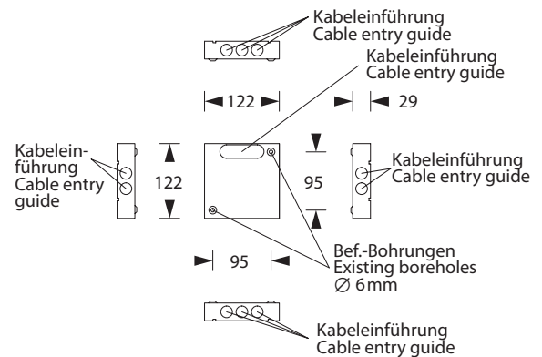
Hinterbaukasten/Back box
